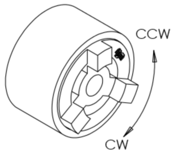
SHAFT INPUT
